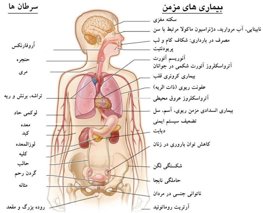
شکل ۱- عوارض سلامتی مرتبط با مصرف تدخینی دخانیات
